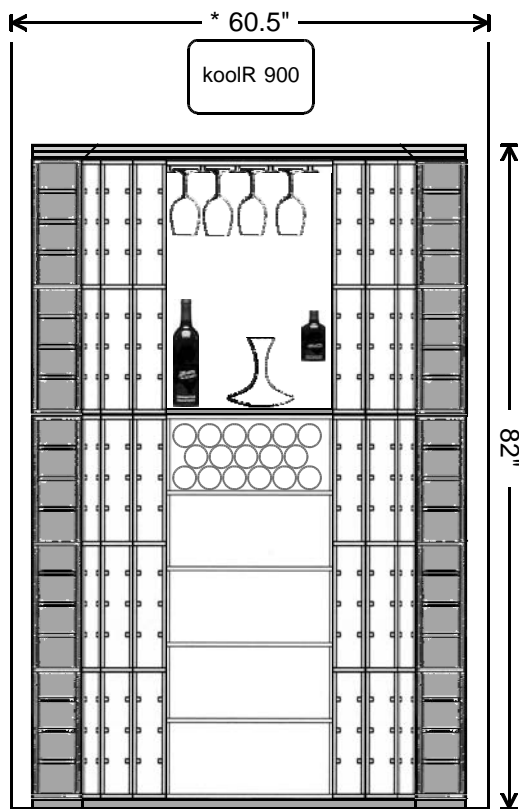
Elevation B
