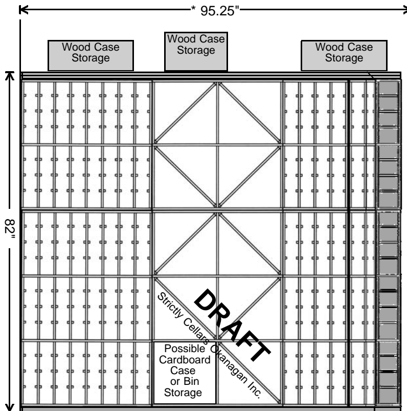
Elevation A
